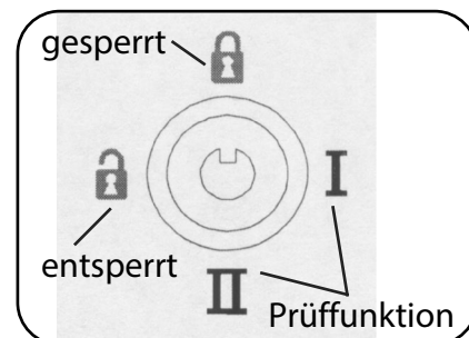
Abb. 8.6.03 – Drehschalterstellungen
